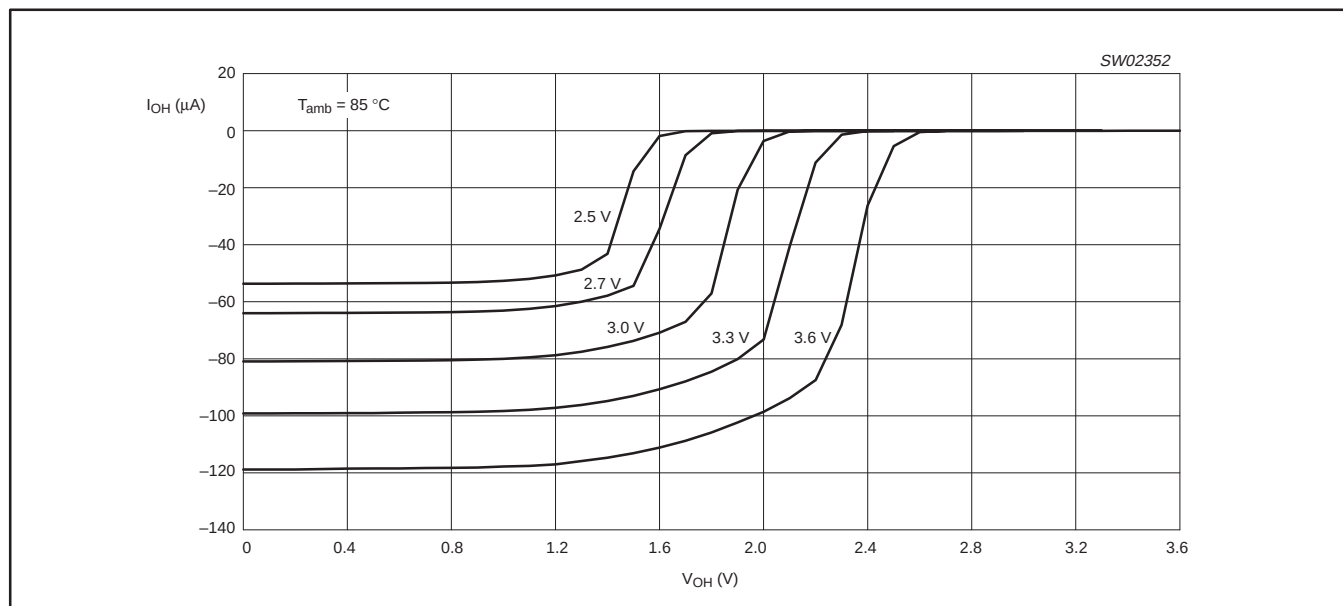
Figure 24. V_{OH} versus I_{OH} ( T_{amb} = 85\text{ °C} )
