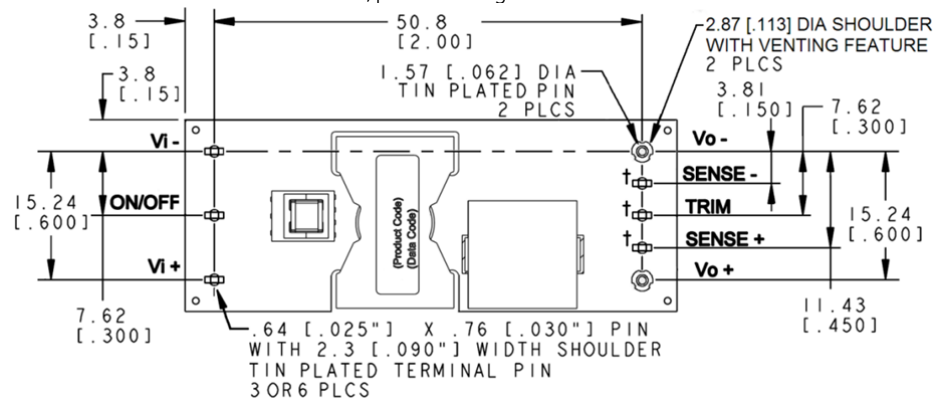
Pin Function 1 Vi(+) 2 ON/OFF 3 Vi(-) 4 Vo(-) 5† SENSE(-) 6† TRIM 7† SENSE(+) 8 Vo(+)
