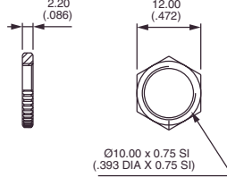
HEX NUT
