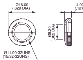
LOCKWASHER
