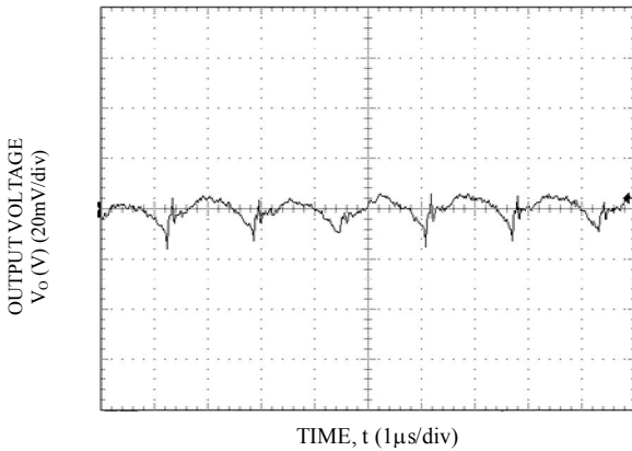
Vo=0.6V, Io = Io,max, Vin=8V
