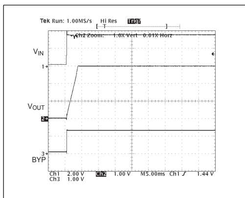
Fast V_{IN} , 1000μF Output Load
