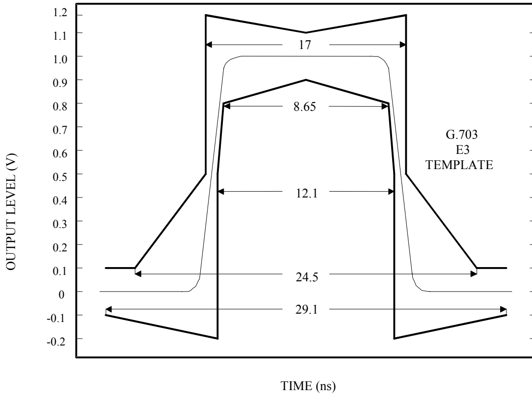
Figure 16-11. E3 Waveform Template
