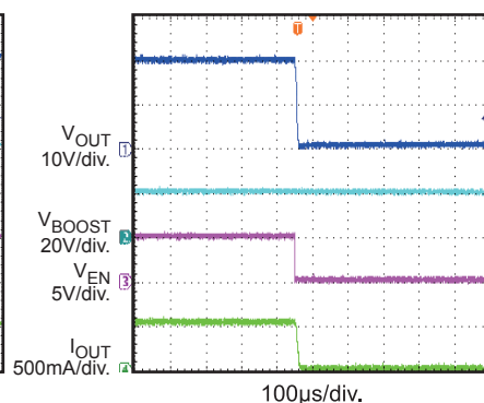
EN Shutdown
