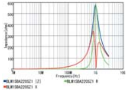
BLM15BA220SZ1
