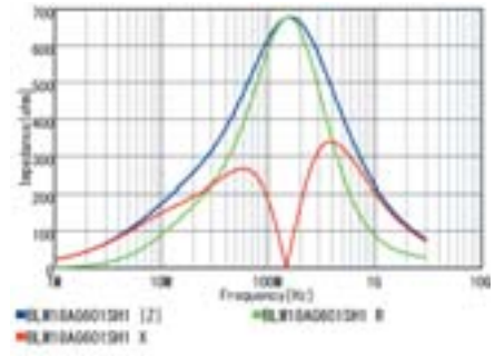
BLM18AG601SZ1/BLM18AG601SH1
