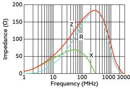
BLL18AG151A2E1H01/BLL18AG151DBE1H01
