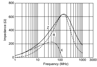
BLM18TG601TN1
