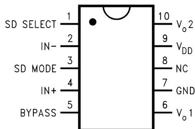
Mini Small Outline (MSOP) Package
