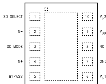
LLP Package
