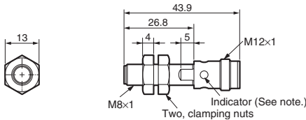
E2A3-S08KS03-M1-□□
