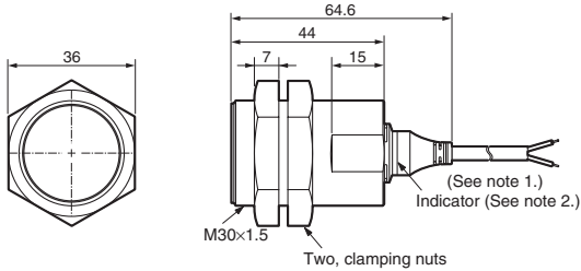
E2A3-M30KS20-WP-□□
