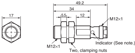
E2A3-M12KS06-M1-□□
