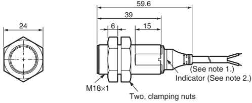
E2A3-M18KS11-WP-□□
