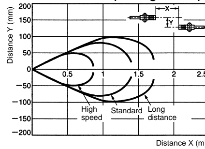
E32-TC200+E39-F1 (Through-beam)
