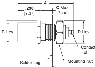
Fig. 2 Plug Receptacle
