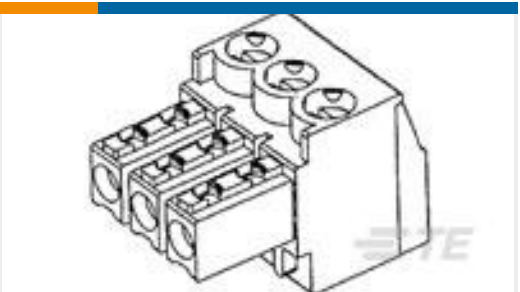
TE Part #284509-3 3P TERMI-BLOK PLUG STACK 3,8
