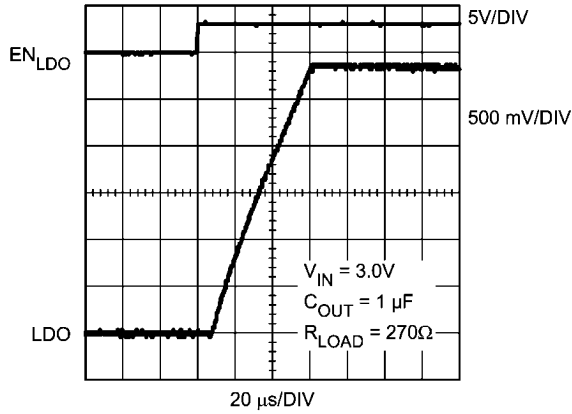
LDO Turn ON (EN LDO = Low to High)
