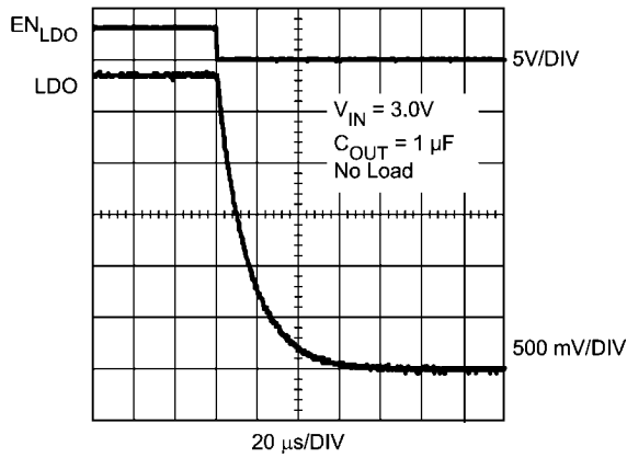
LDO Turn OFF (EN LDO = High to Low)
