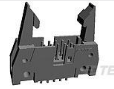
TE Part #5499206-8 A/L UNIV HDR 34P VERT LAT
