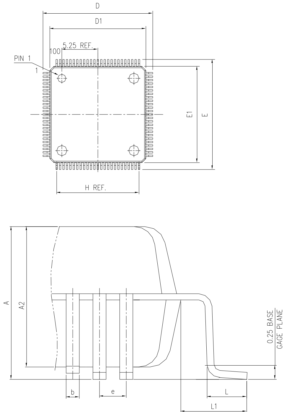
图 17 LQFP100 封装图
