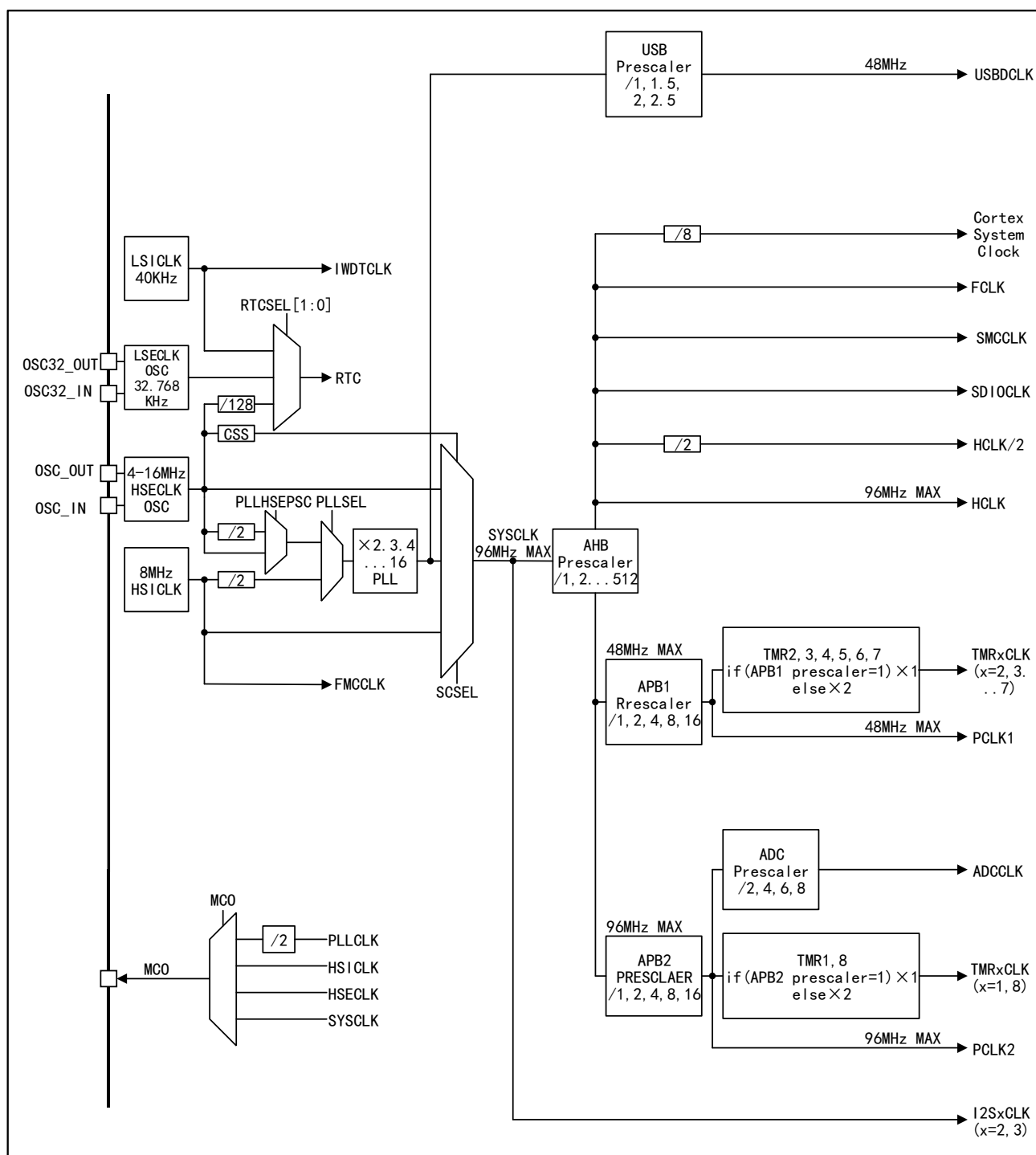
图 7 APM32F103xC 时钟树
