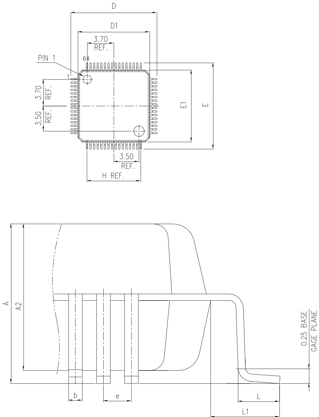
图 20 LQFP64 封装图
