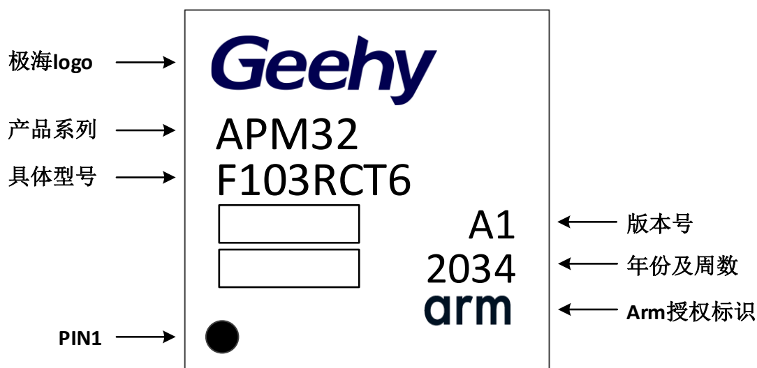
图 22 LQFP64-64 引脚，10×10mm 封装标识
