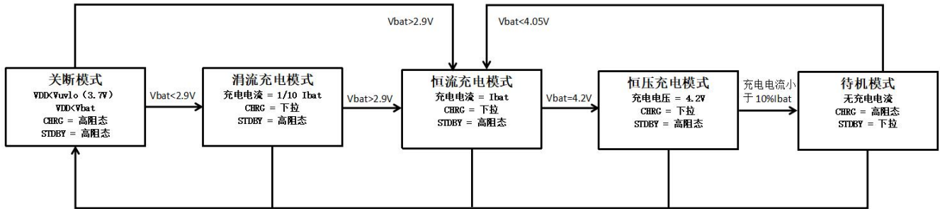
图 1 典型充电循环的状态图。
