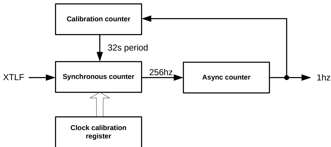
图 36-2LTBC 结构框图
