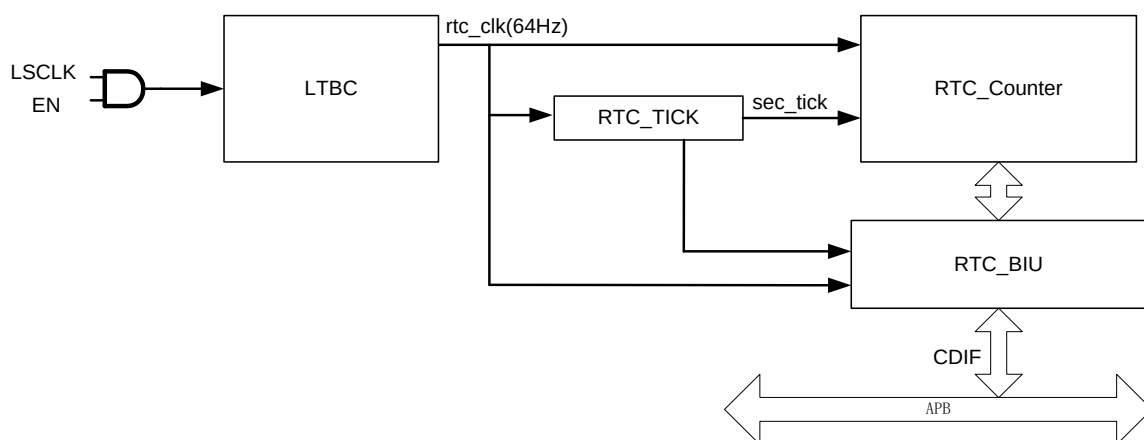
图 35-1 RTC 结构框图
