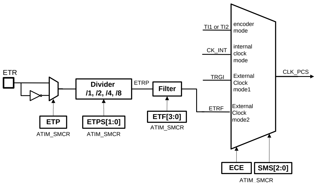
图 29-21 外部触发输入框图
