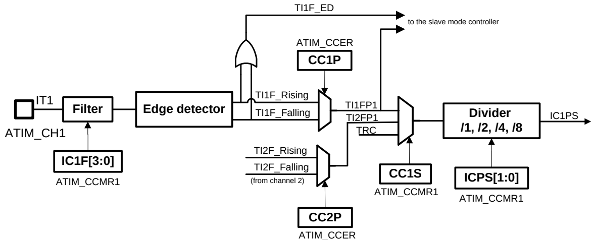
图29-24捕捉/比较通道(通道1输入部分)
