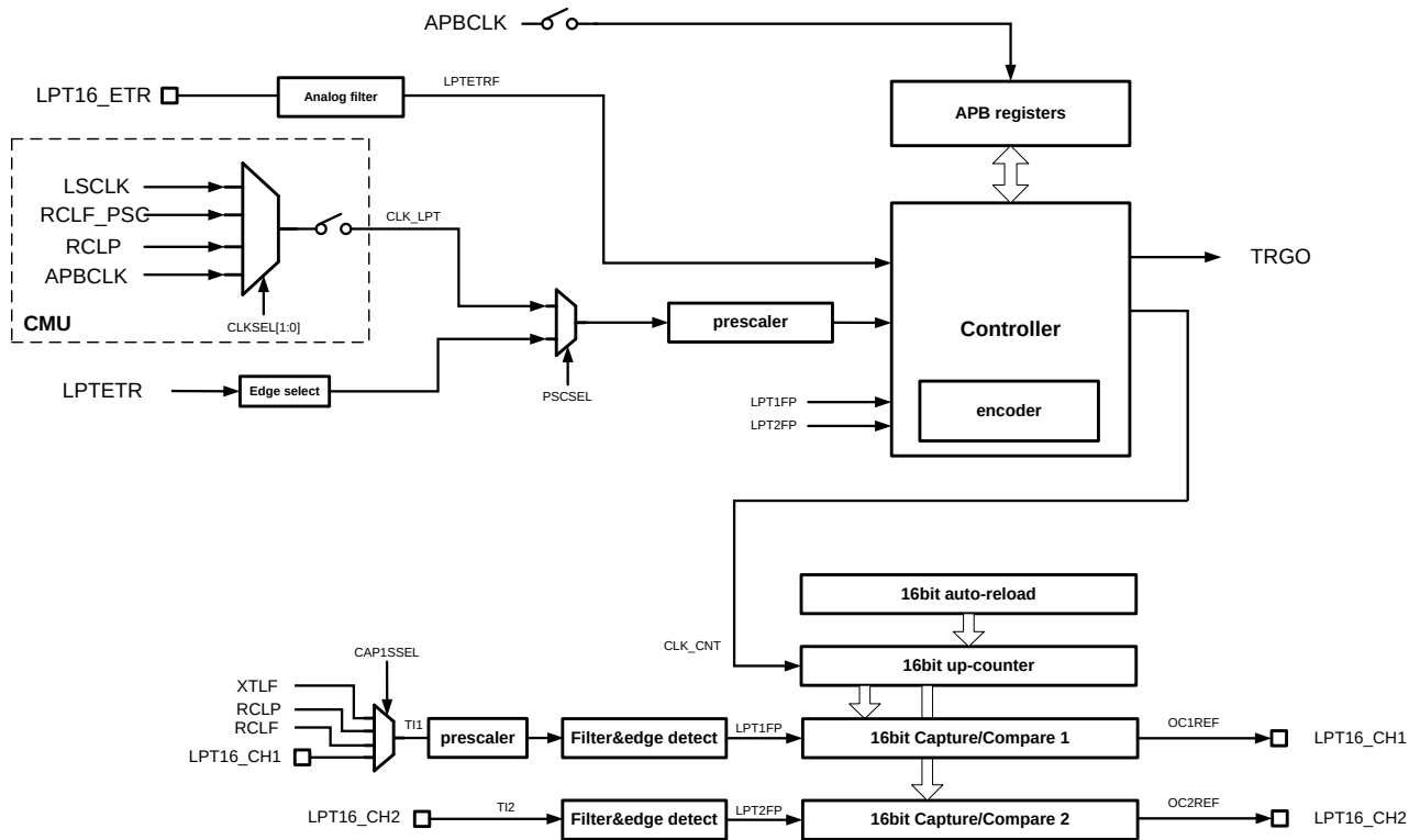
图 34-1 LPTIM16 结构框图
