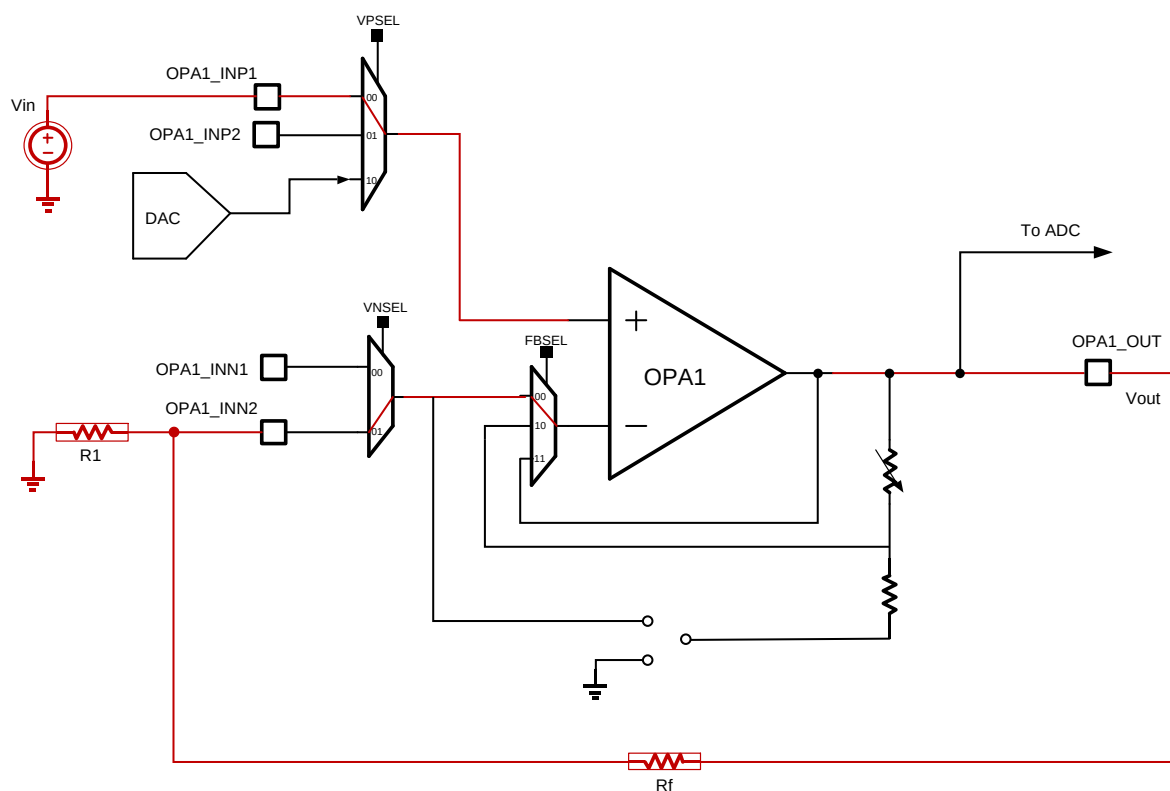
图 18-3OPA 非反相放大
