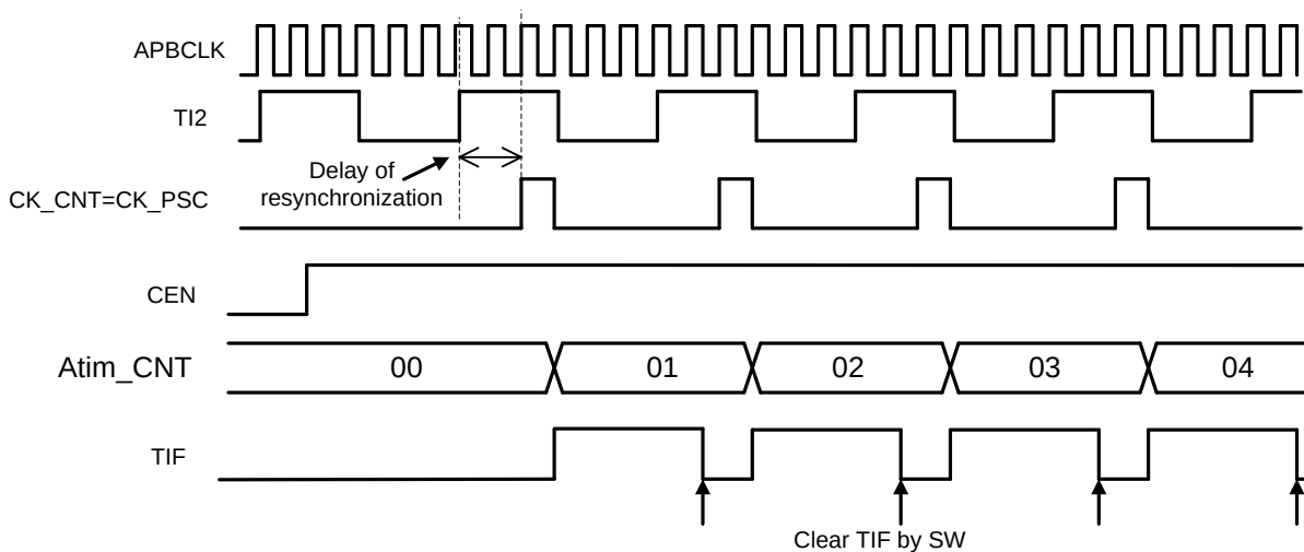
图 29-20 外部时钟模式 1 下的时序
