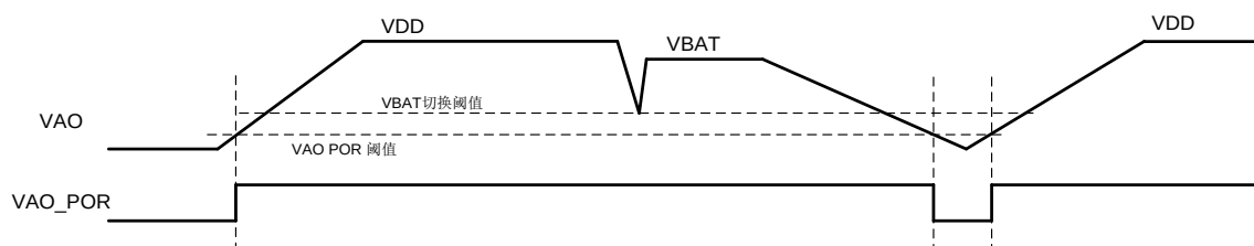
图 8-2 VAO 上下 RTCB 电复位示意图
