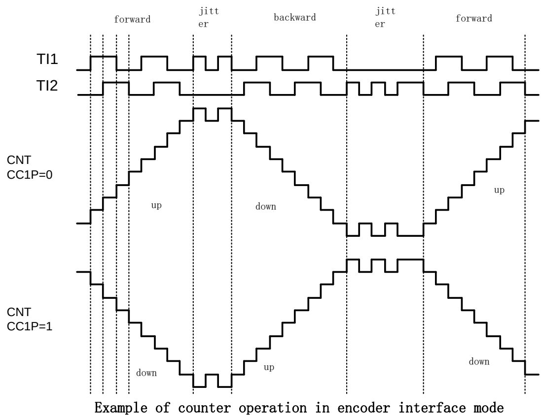
图30-32编码器模式下的计数器操作实例
