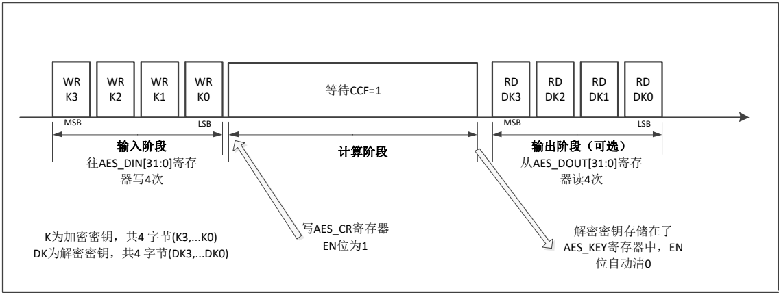
图 16-14 模式 2 示意图
