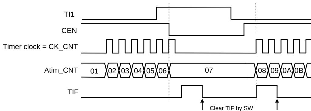
图29-41门控模式下的时序
