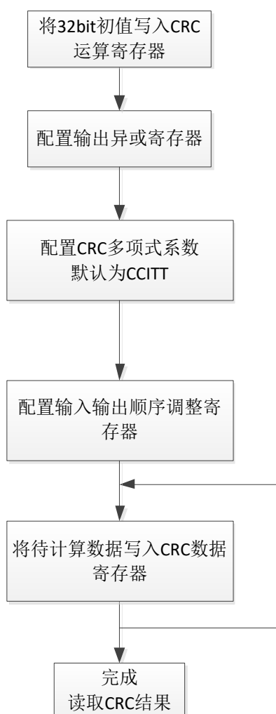
图 28-1 CRC 运算流程图
