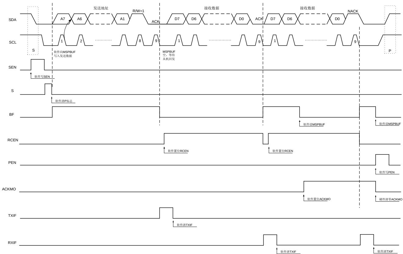
图 21-12 I2C 从 7 位地址从机读取数据流图
