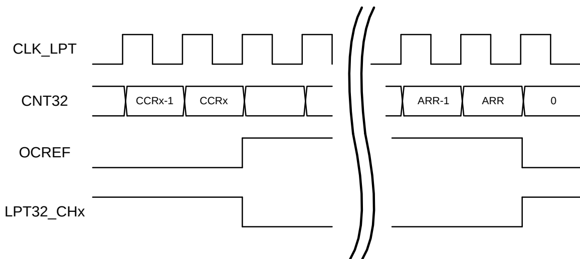
图 33-5 PWM 输出
