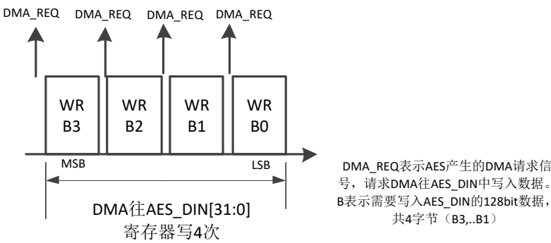
图 16-18 输入时 DMA 请求和数据传输示意图
