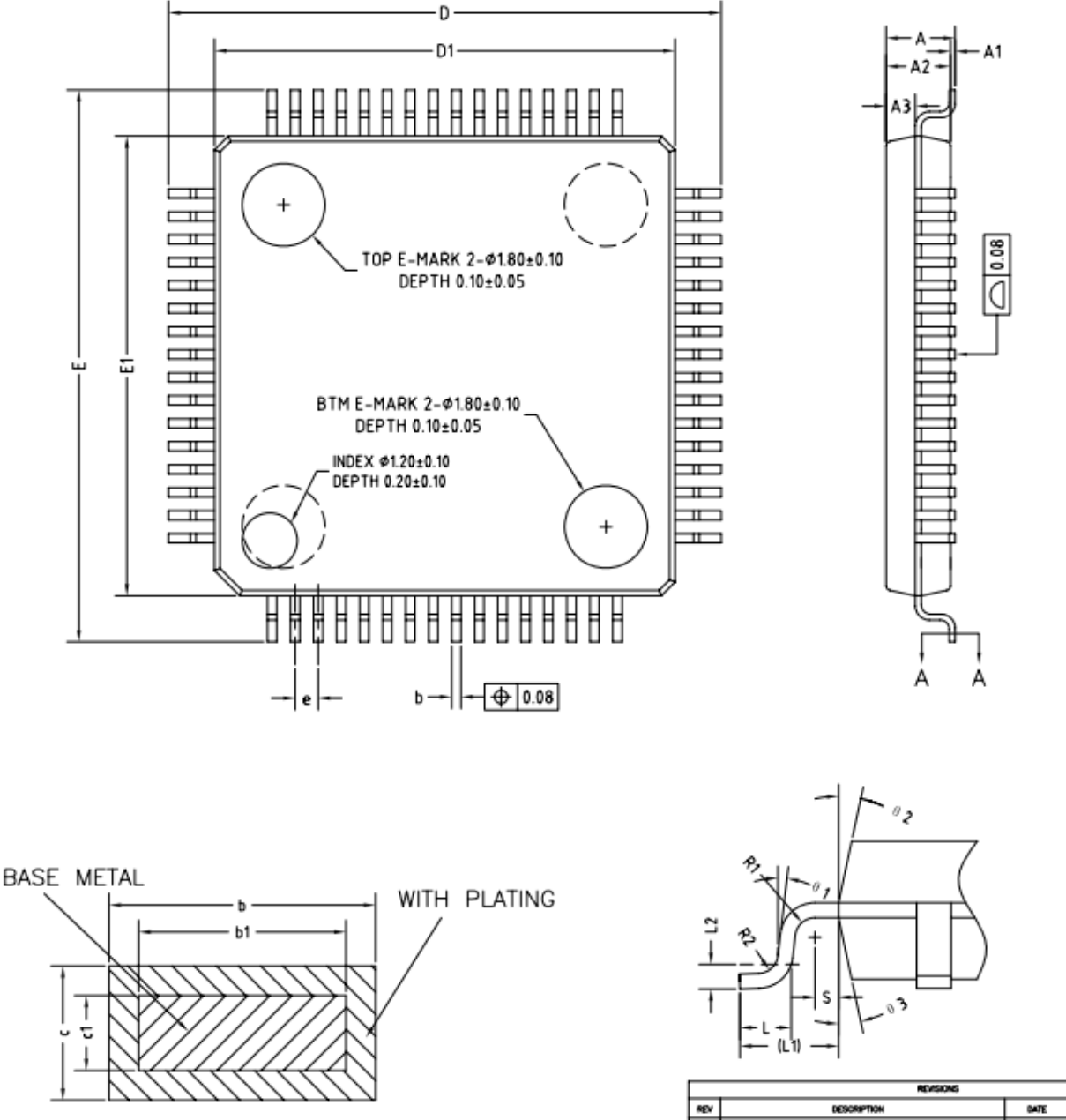
图 2-6LQFP64 封装尺寸图
