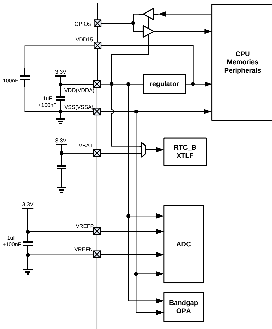
图 3-1FM33LG0xx 测试条件
