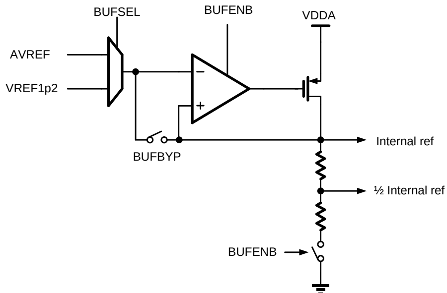
图 19-2 比较器内建基准缓冲器
