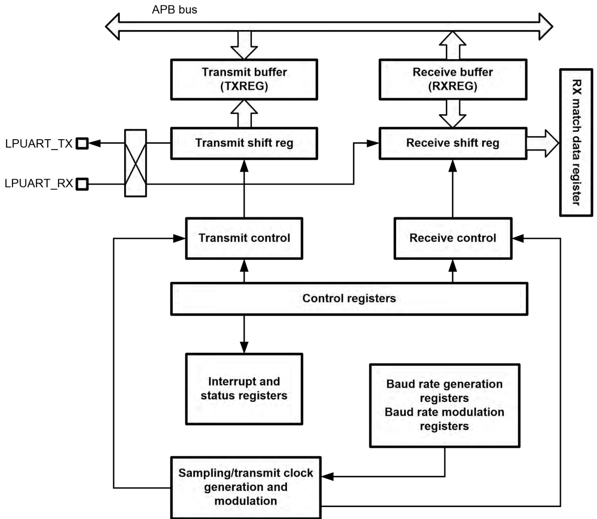
图 22-1 LPUART 结构框图
