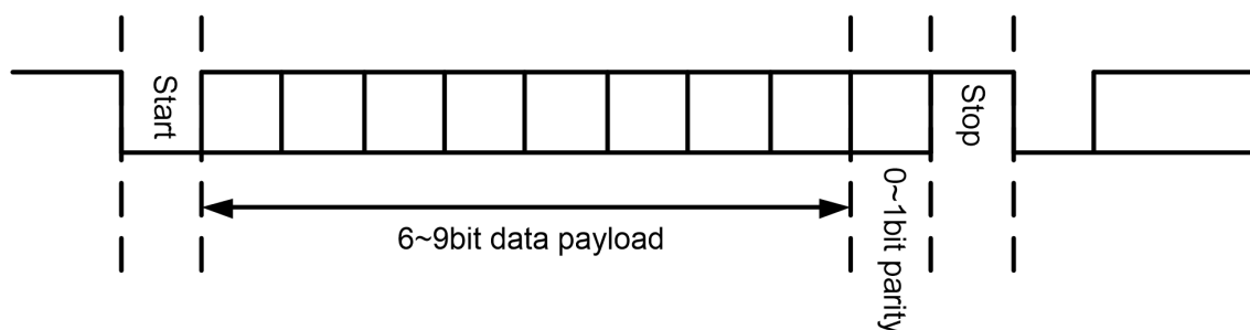
图 20-2 UART 字符描述
