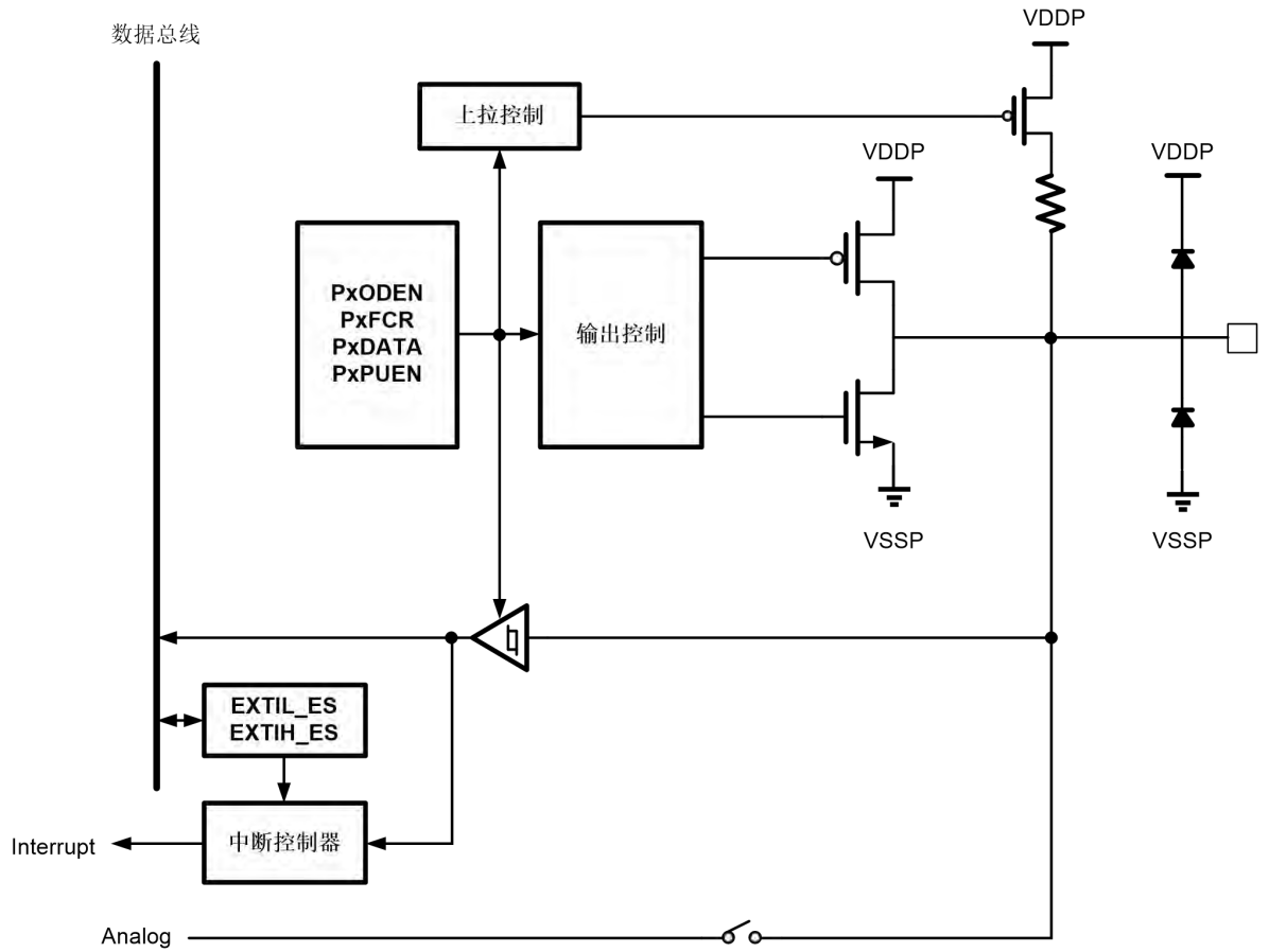
图 34-1 普通 GPIO 结构框图
