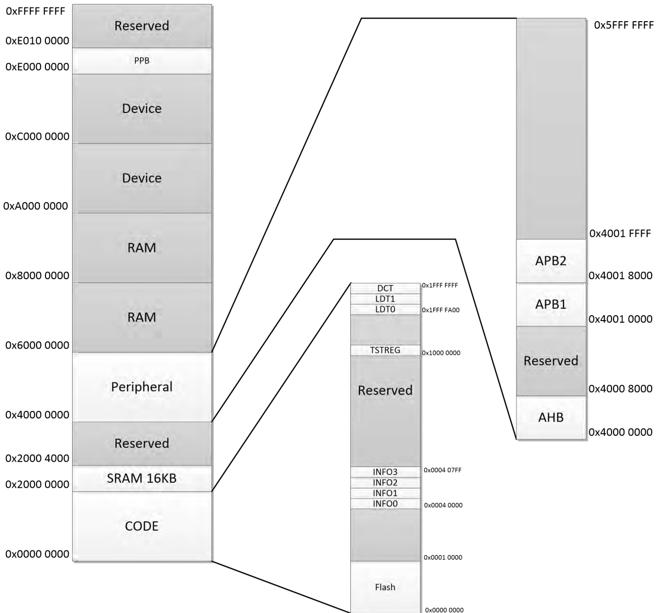
图 7- 3FM33LE01x 总线地址
