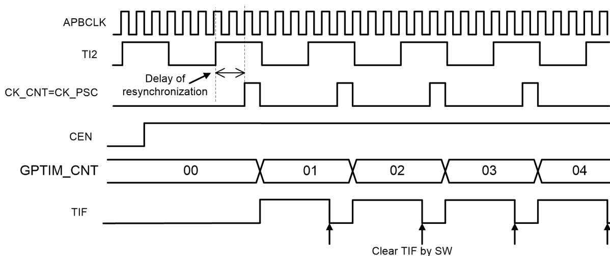
图 28-19 外部时钟模式 1 下的时序
