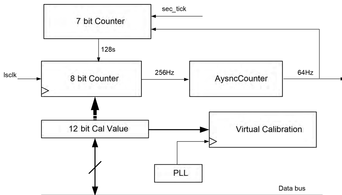
图 31-2LTBC 结构框图
