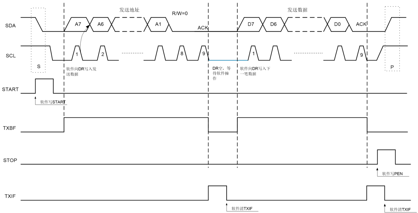
图 18-9 I 2 C 主机对 7 位地址从机发送数据流图
