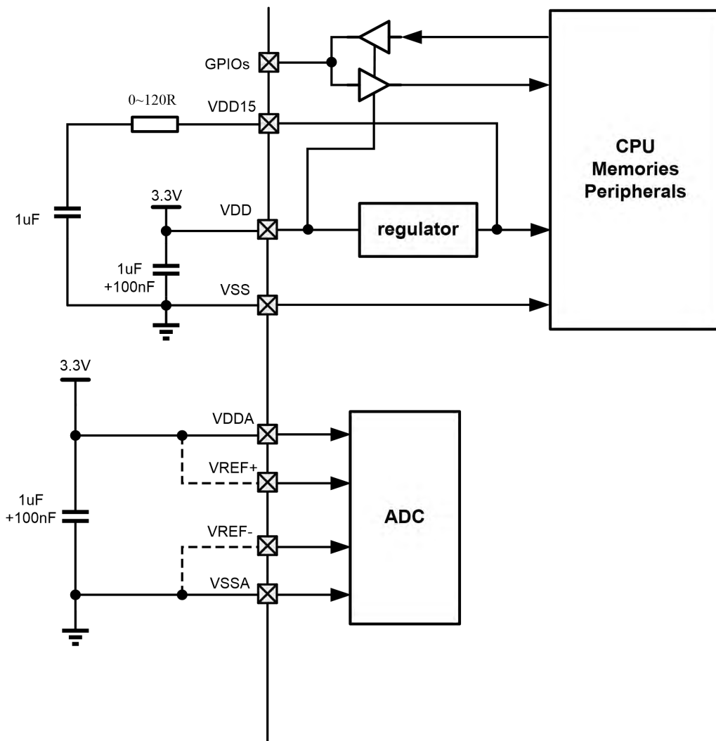
图 3-1 FM33LE0 供电方案
