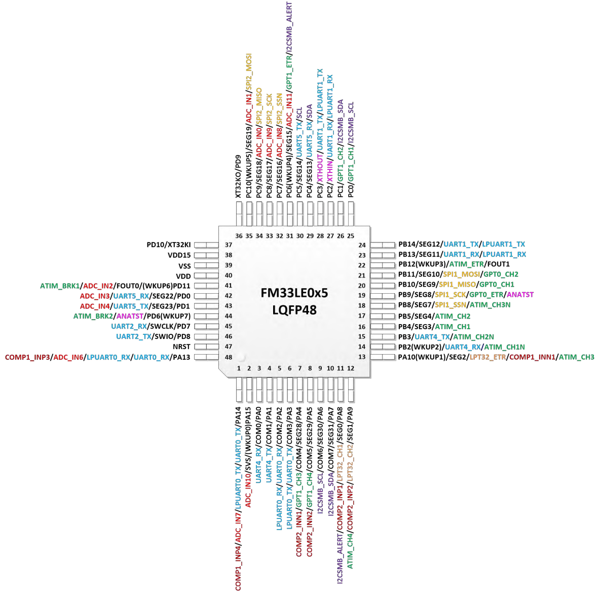
图 2-2FM33LE0x5 LQFP48 封装图
