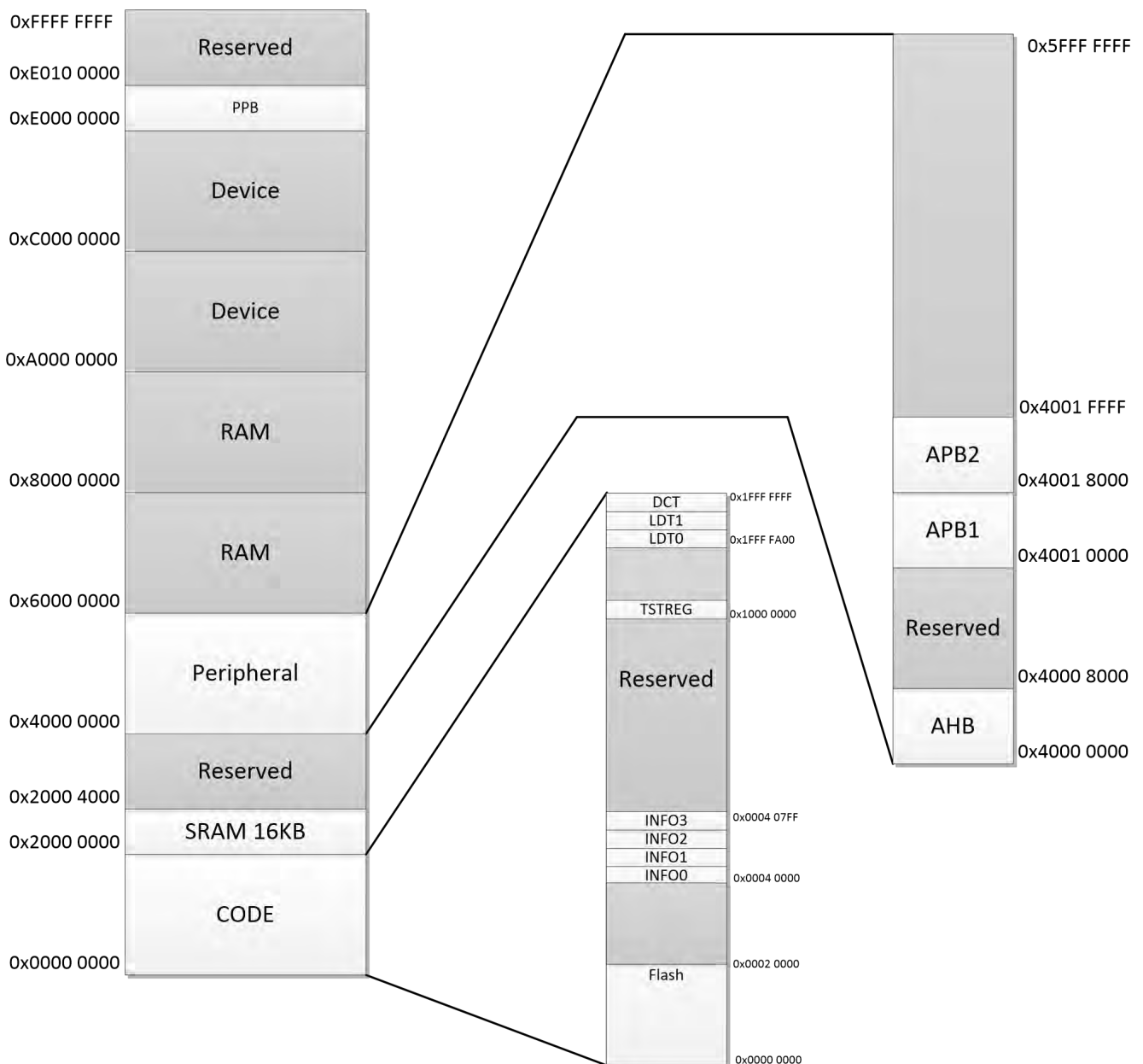
图 7-2FM33LE02x 总线地址
