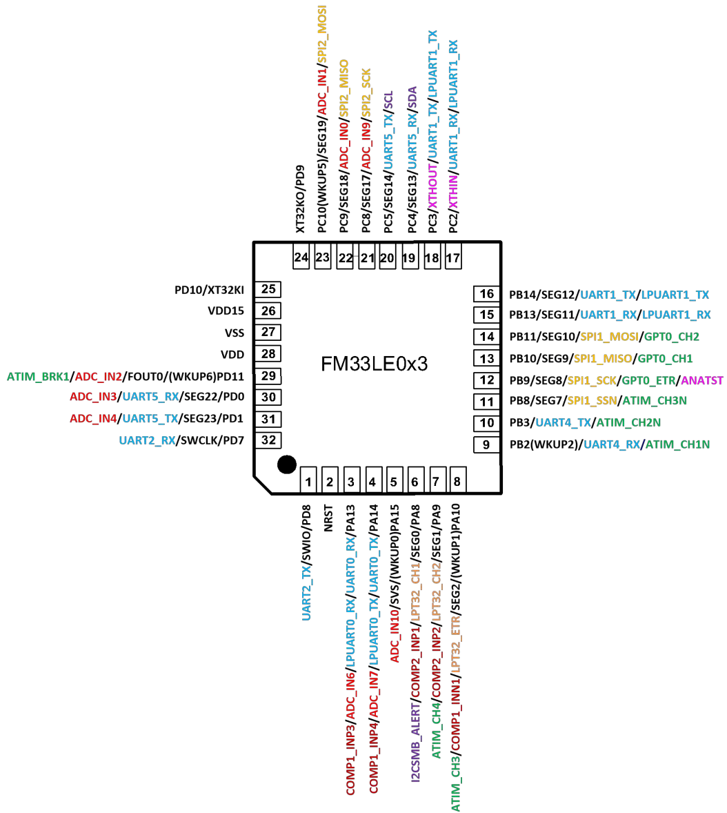
图 2-5 FM33LE0x3 QFN32 封装图
