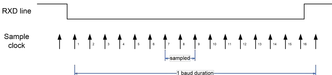
图 20-3 位接收采样
