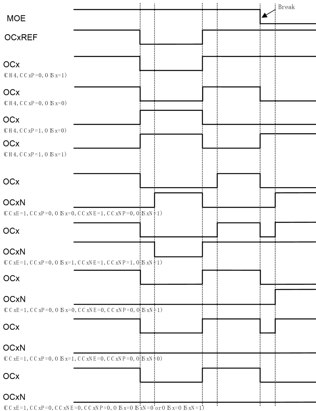
图27-35响应刹车的输出
