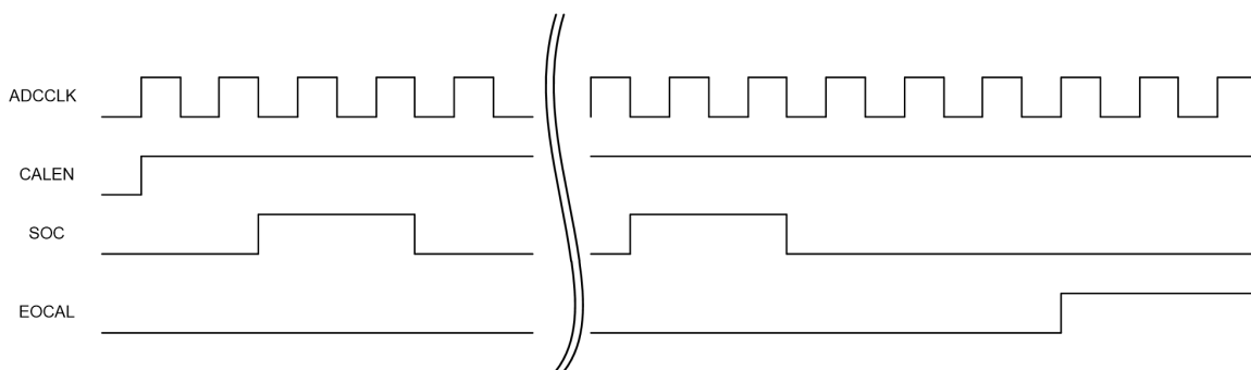
图 33-2 ADC 校准时序
