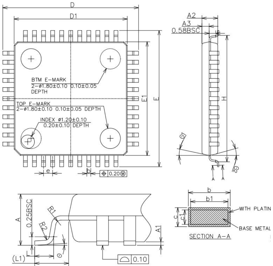
图 2-8LQFP44 封装尺寸图
