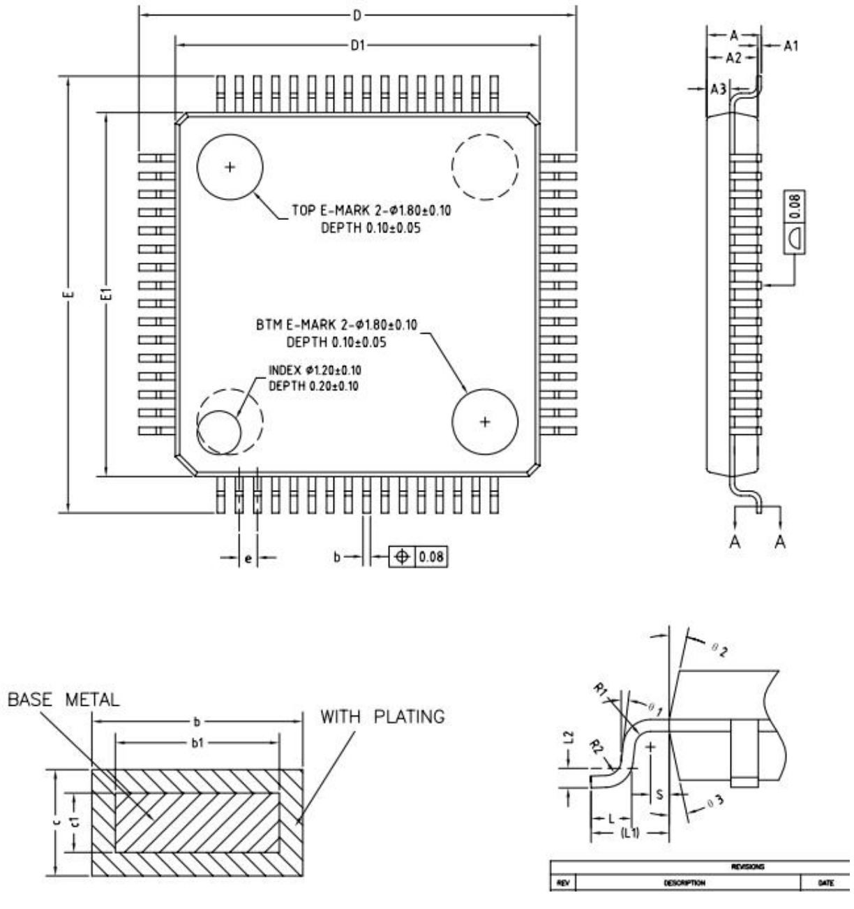
图 2-6 LQFP64 封装尺寸图
