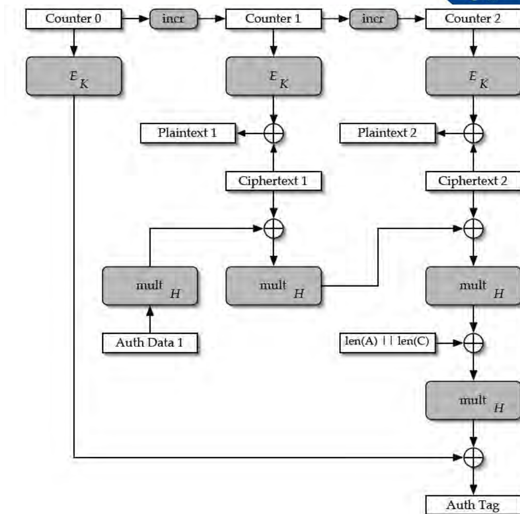
图 14-10 GCM 解密流程
