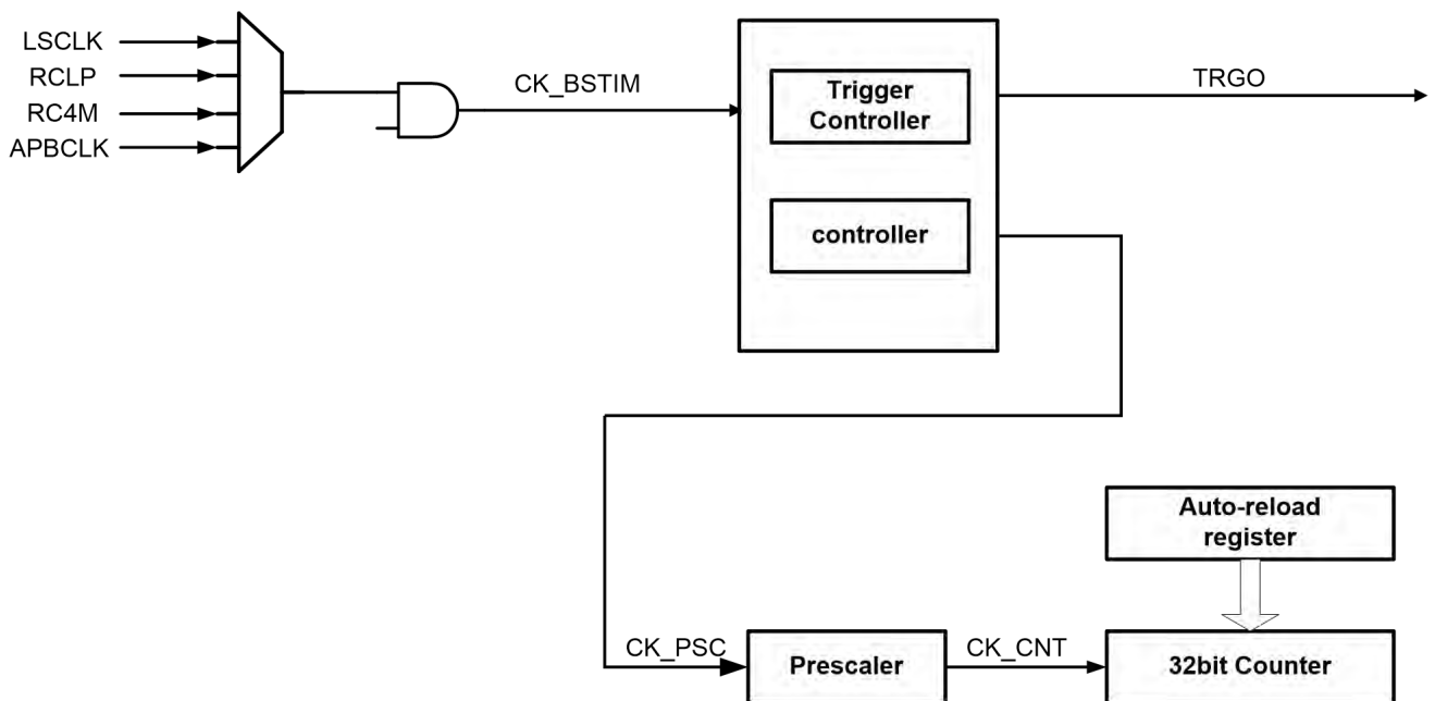
图29-1 BSTIM32结构框图
