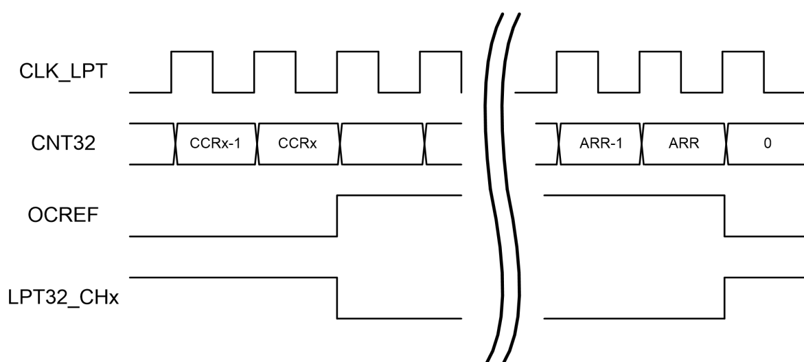
图 30-5 PWM 输出
