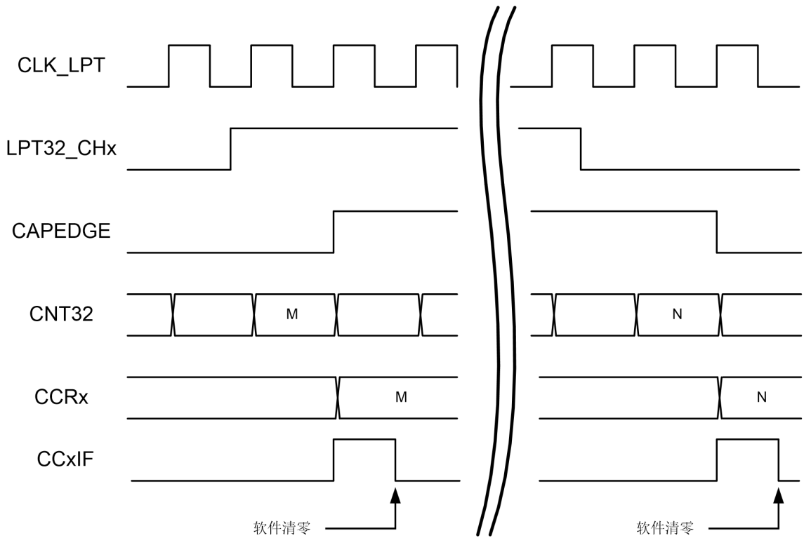
图 30-6PWM 输出
