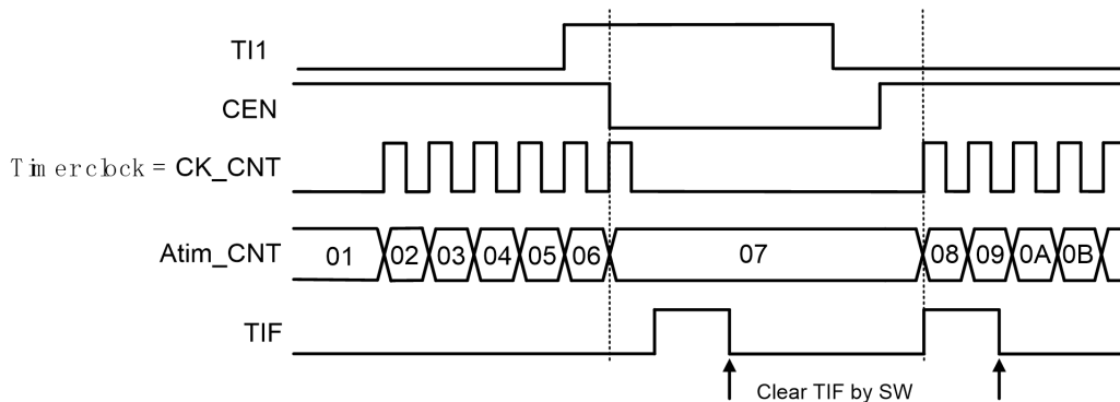
图27-41门控模式下的时序
