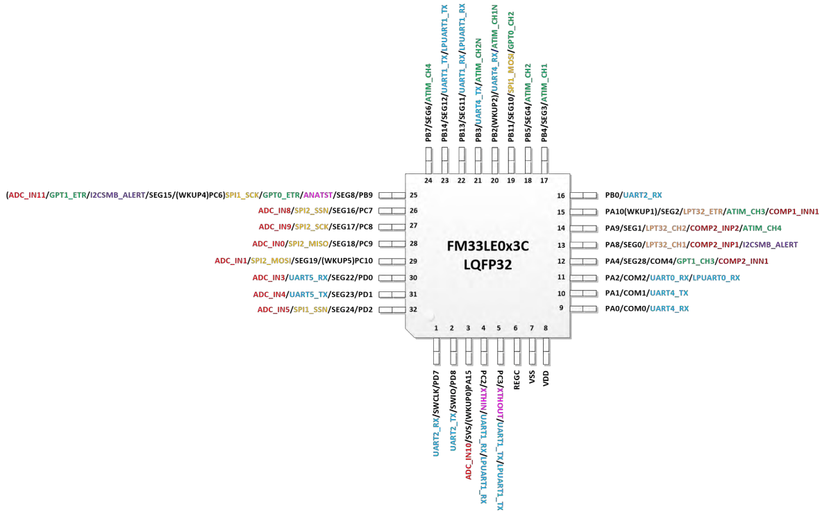
图 2-4FM33LE0x3C LQFP32 封装图
