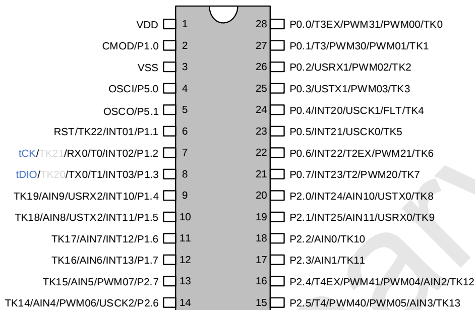
SC95F8673 管脚配置图 适用于 SOP28、TSSOP28 封装
