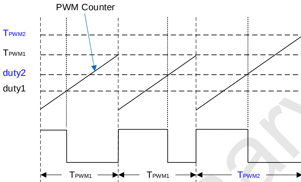
边沿对齐的 PWM
