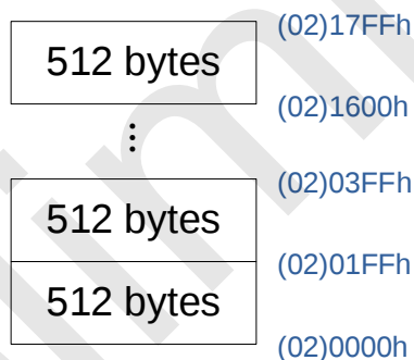
SC95F867X EEPROM Sector 分区示意
