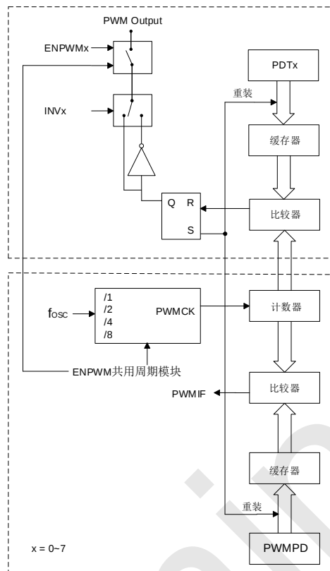
SC95F867X PWM 结构框图
