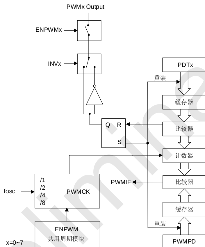
SC95F867X PWM 独立模式框图
