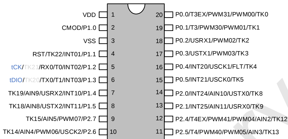
SC95F8672 管脚配置图 适用于 SOP20、TSSOP20 封装
