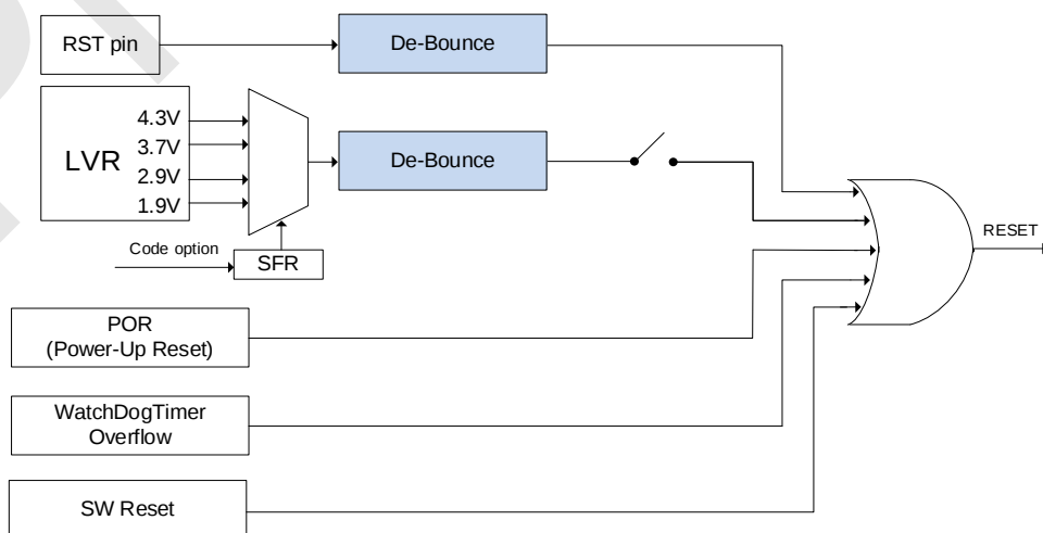
SC95F867X 复位电路图
