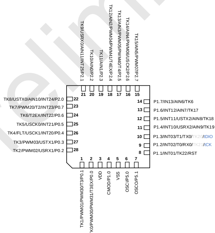
SC95F8673 管脚配置图 适用于 QFN28 封装
