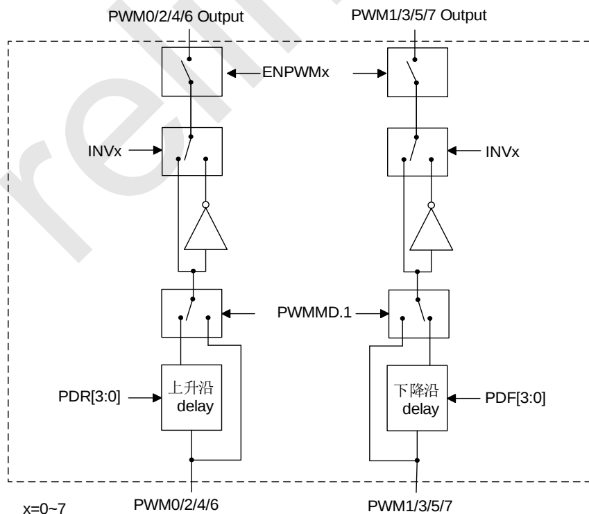
SC95F867X PWM 互补模式框图
