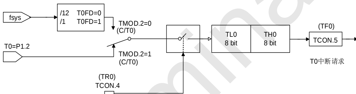
定时器/计数器工作模式 1: 16 位定时器/计数器
