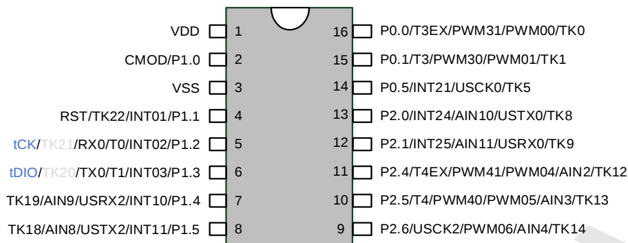
SC95F8671 管脚配置图 适用于 SOP16 封装
