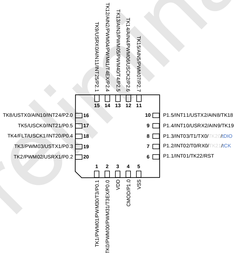
SC95F8672 管脚配置图 适用于 QFN20 封装
