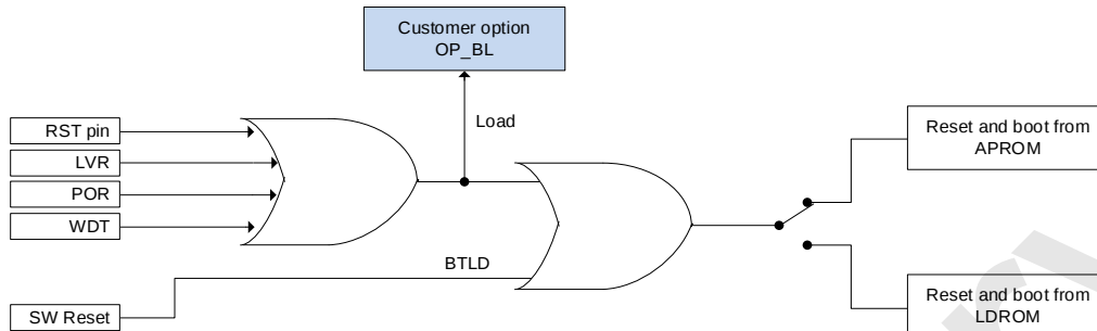
SC95F867X 复位后启动区域切换示意图
