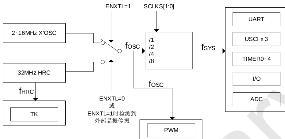
SC95F867X 内部时钟关系
